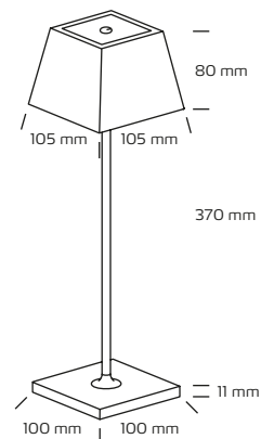
*Tegningen er ikke målfast
